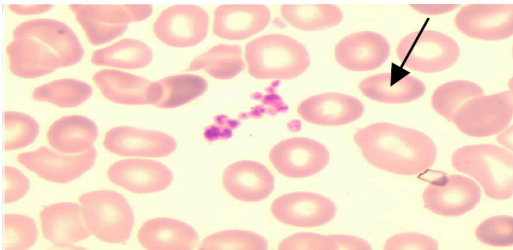
Figure 2 : Agrégats plaquettaires
